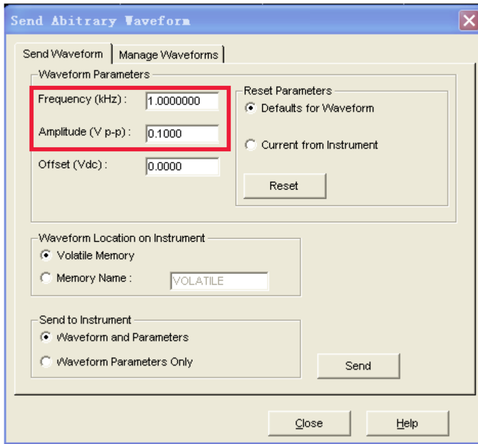
Figure 9. Waveform parameter setup
